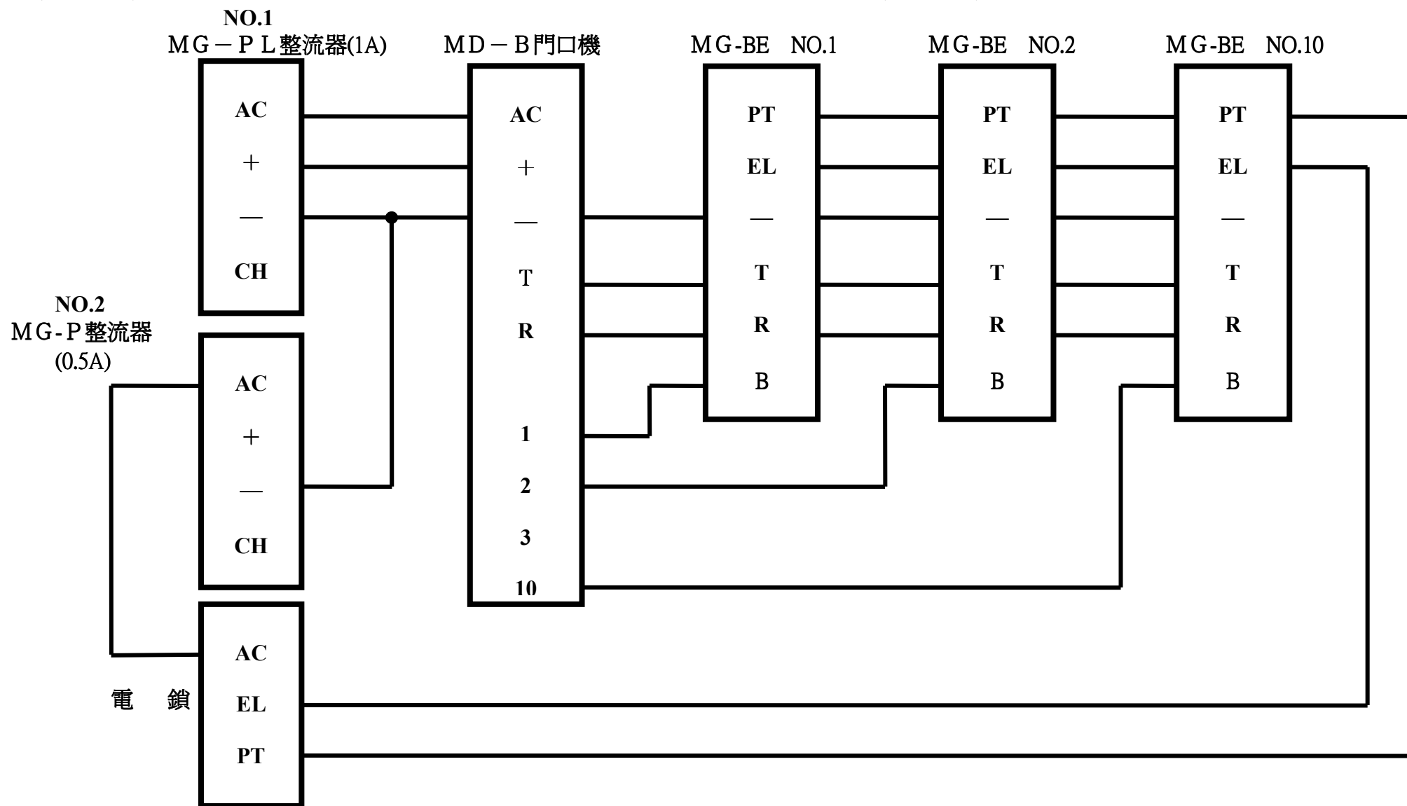
MG-B E 公寓式對講機配接圖(雙電源)
